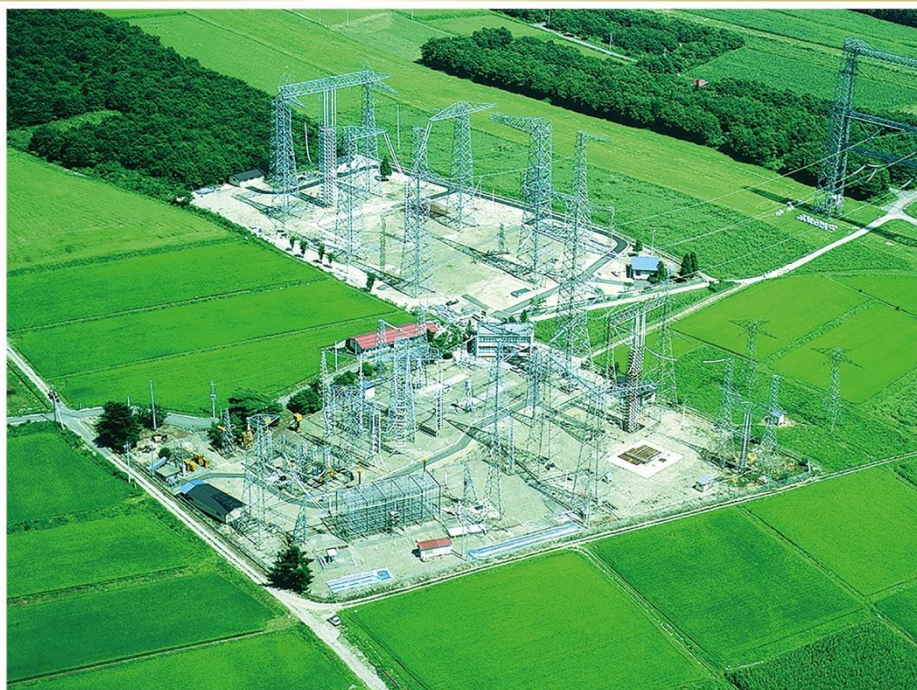
写真：那須塩原市 塩原実験場は世界最大級の雷試験設備
